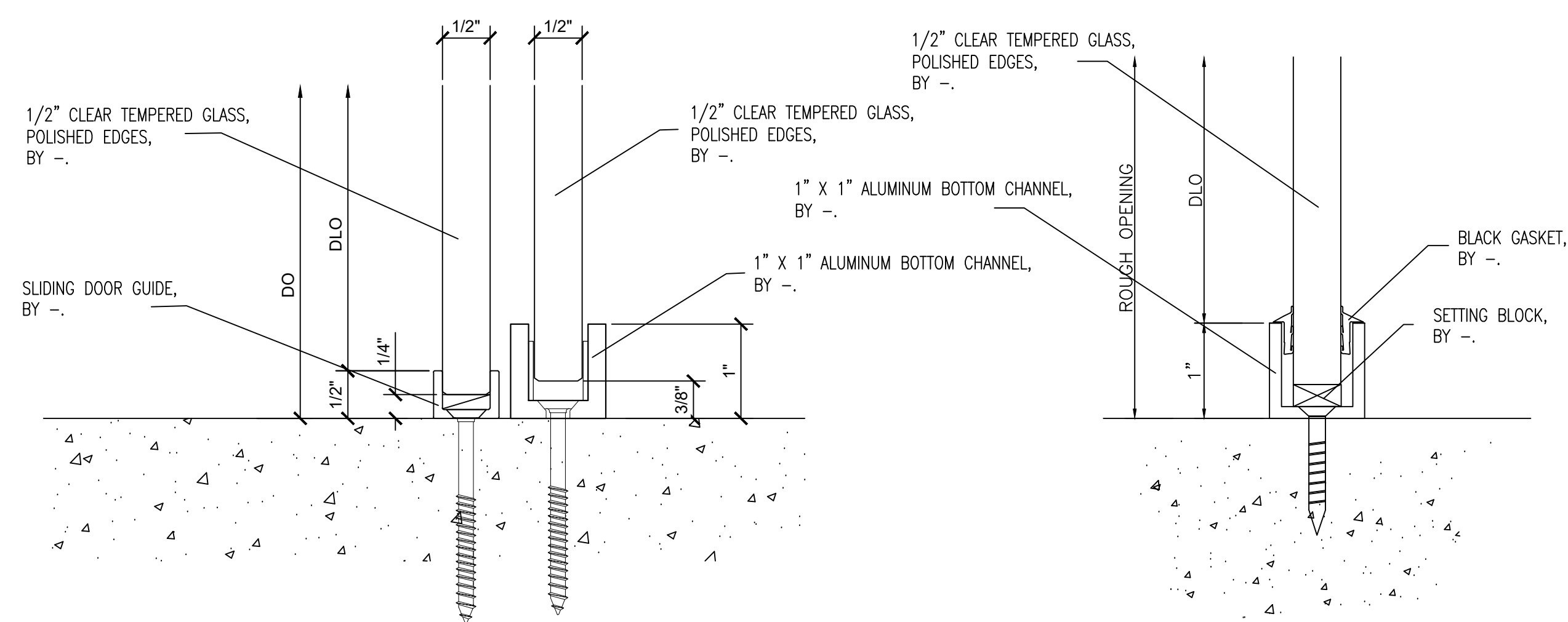
2 SECTION CUT ● SLIDING DOOR GUIDE
